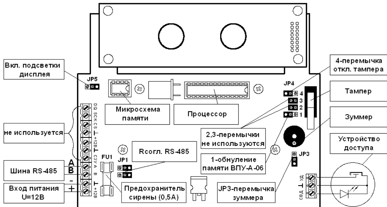
Рисунок 2 - Внешний вид клавиатуры ВПУ-А-06 со снятой задней крышкой
