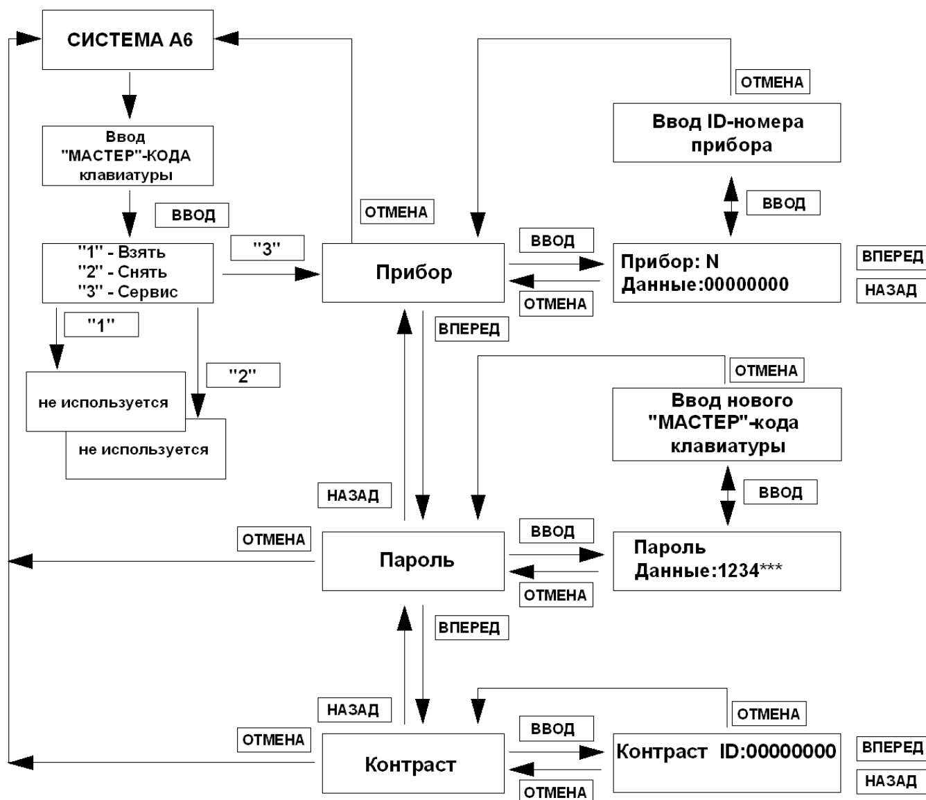
Рисунок 9 - Блок схема работы ЖКИ клавиатуры ВПУ-А-06 в режиме «Система»
