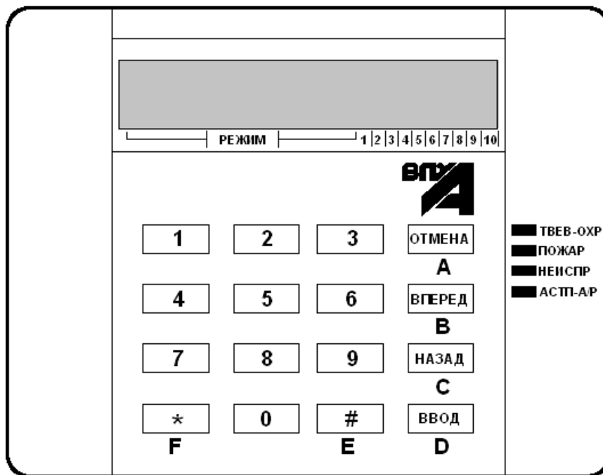
Рисунок 1 – Внешний вид выносной панели управления ВПУ-А-06 (ВПУ-А-16)
